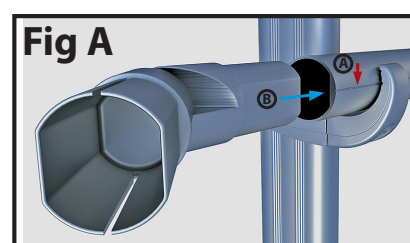
Fig A Les lisses doivent être montées à l'horizontal selon le repère (A) pour le montage jonctions (B).
