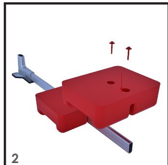
2 Fixez les plots avec la visserie fournie (un garde-corps sur deux).
