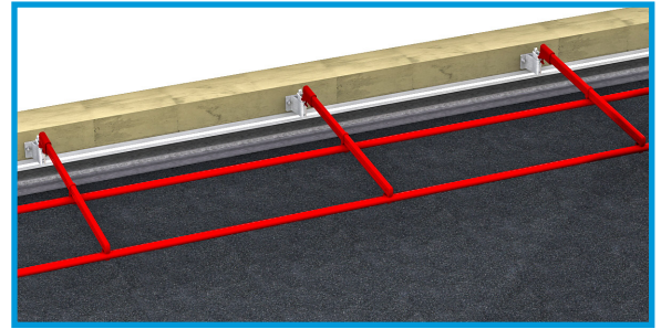
3 Répéter l'opération sur chacun des montants du tronçon, puis rabattre l'ensemble au sol.
