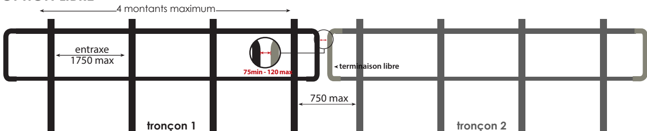
1 Assembler la jonction avec les 2 mains courantes.
