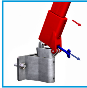
2 Tirer le papillon et basculer légèrement le montant.
