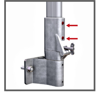
4 Serrer les 2 vis BTR.
