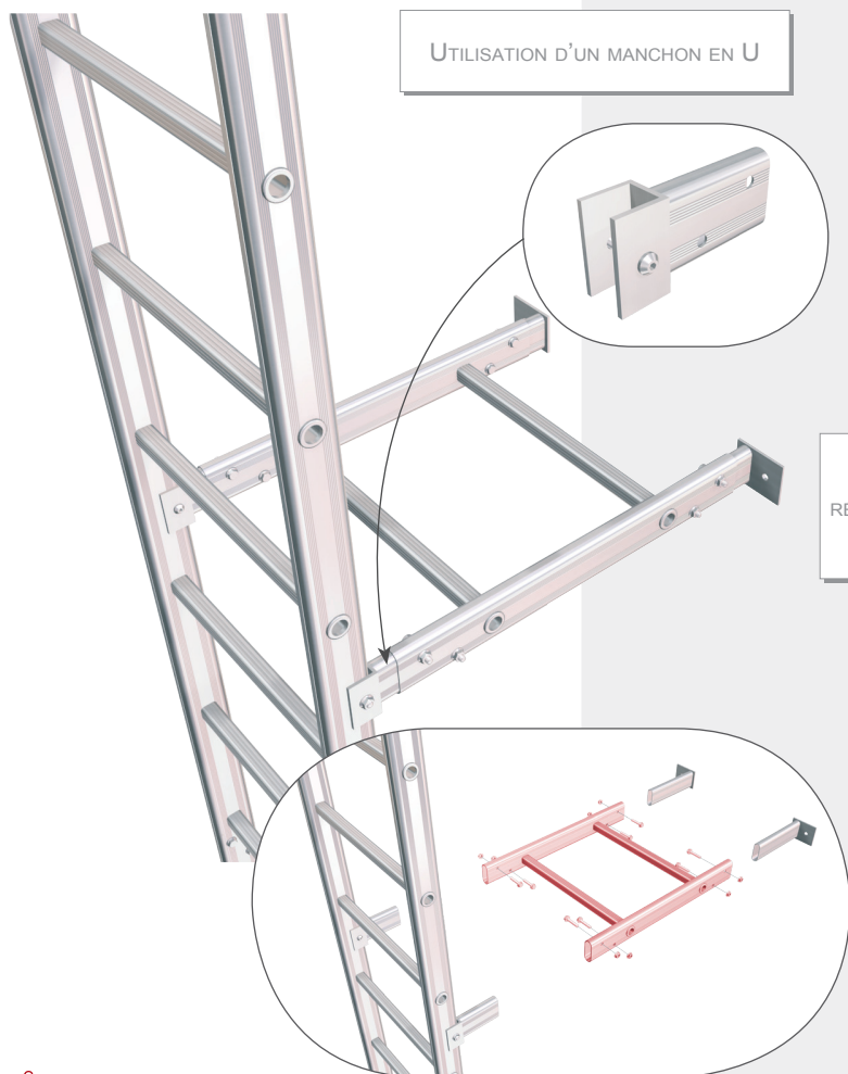
PATTES ÉCARTEUR
